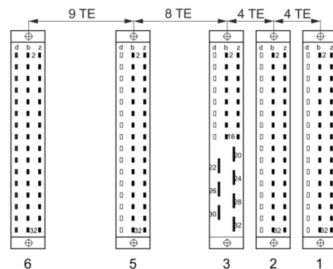
Lage der Federleisten PAN-D
