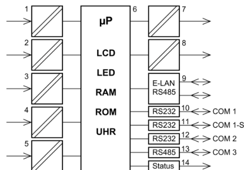
Funktionen des Reglers REG-D™
