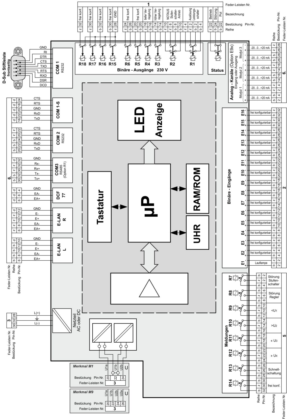
Blockschaltbild PAN-D Merkmal D2 / D3 / D4 / D5
