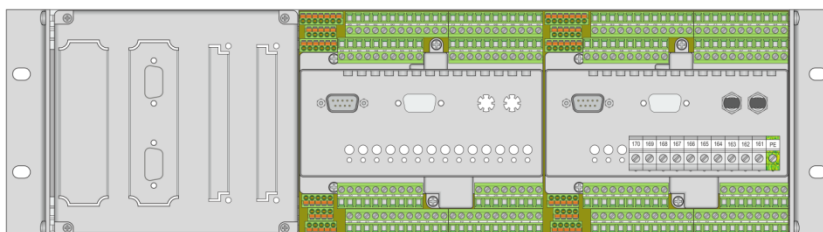
Baugruppenträger 84 TE mit Phoenix Steckschraubklemmen Rückansicht - Merkmal B93
