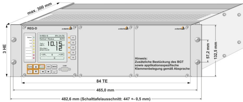
Baugruppenträger 84 TE Frontansicht - Merkmal B92/B93/B95
