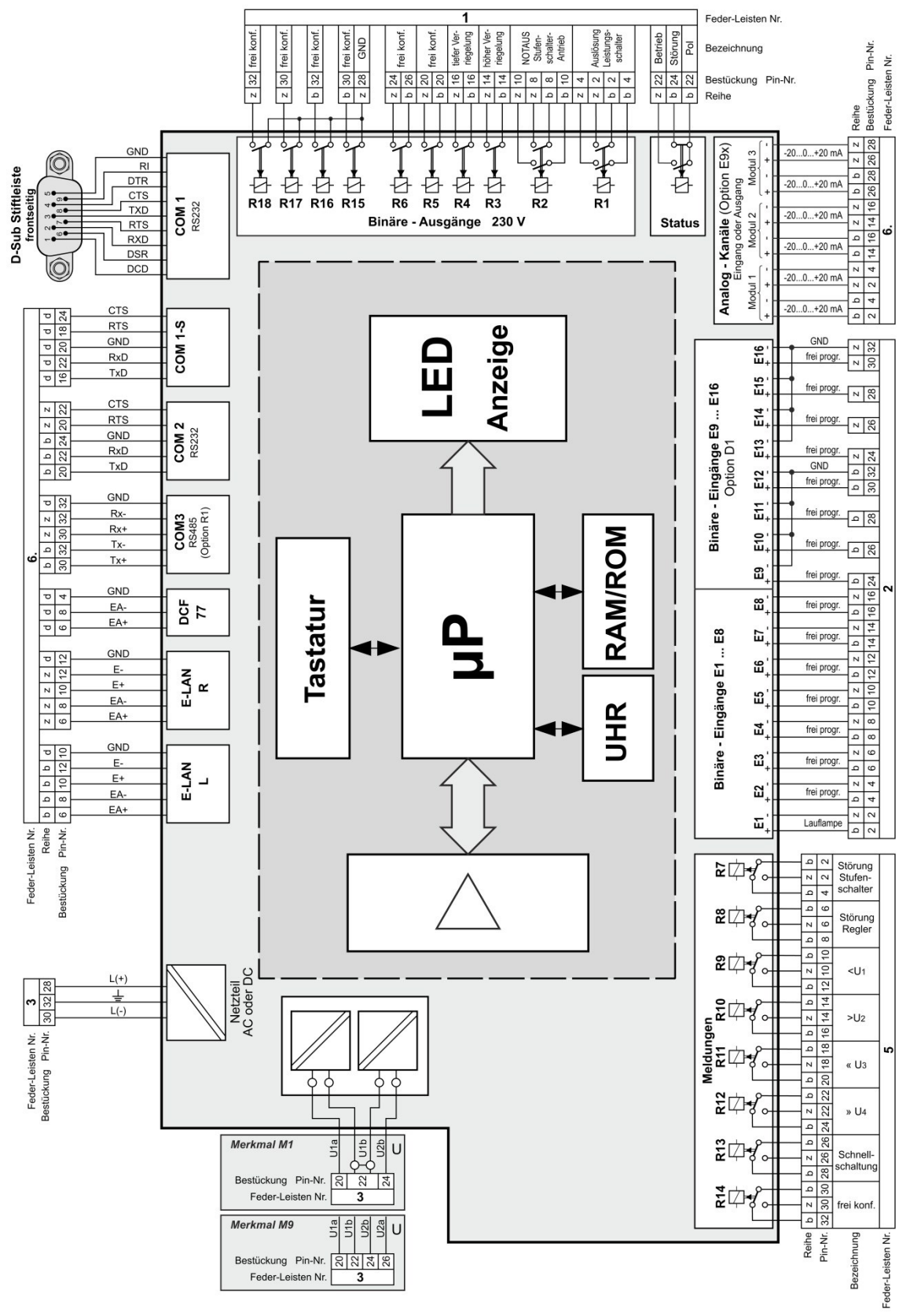
Blockschaltbild PAN-D Merkmal D1
