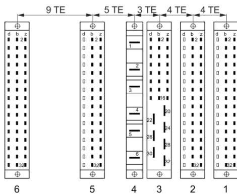
Lage der Federleisten REG-D™
