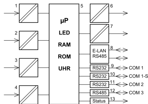
Funktionen der Überwachungseinheit PAN-D
