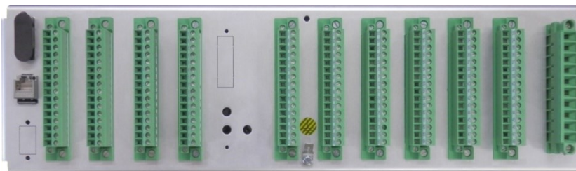
Baugruppenträger 84 TE Rückansicht mit Schraubklemmen - Merkmal B92
