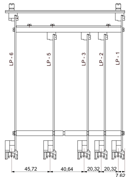
Lage der Messerleisten PAN-D
