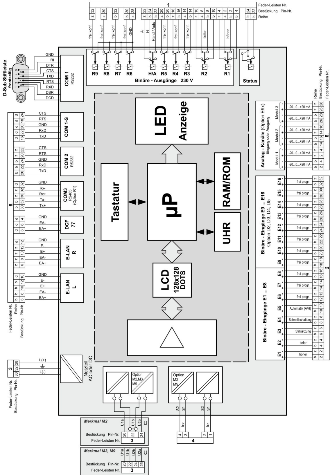
Blockschaltbild REG-D™ Merkmal D2 / D3 / D4 / D5
