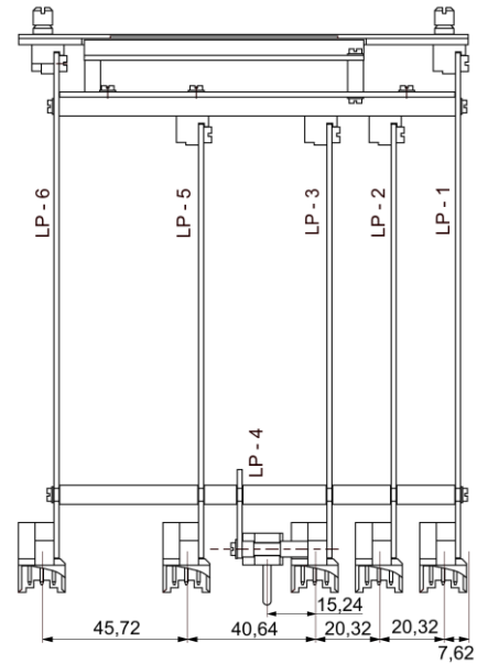
Lage der Messerleisten REG-D™
