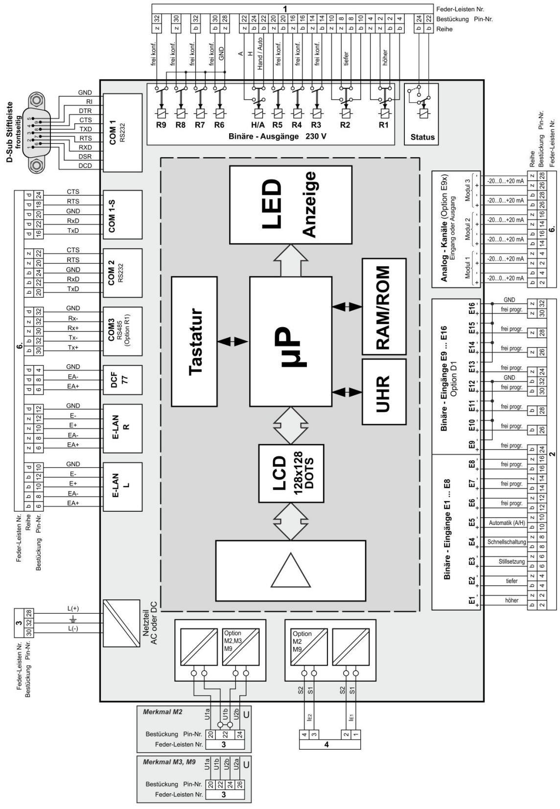
Blockschaltbild REG-D™ Merkmal D1
