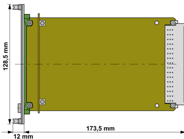
Steckbaugruppe REG-D™ / PAN-D 28 TE - Merkmal B01
